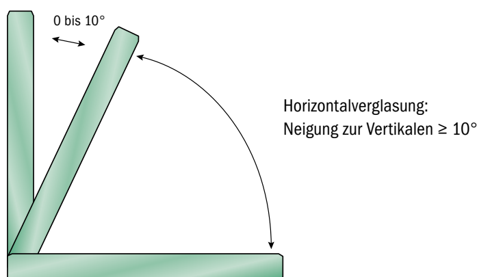
Abb. 4: Definition von Horizontalverglasung nach DIN 18008 (Nach der EN 13830 werden Horizontal- zu Vertikalverglasungen bei 15° unterschieden.)
