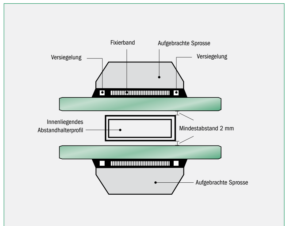
Abb. 5: Beispiel für Wiener Sprosse
